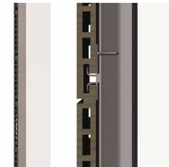
3.1 Dettagli posa orizzontale con clip
