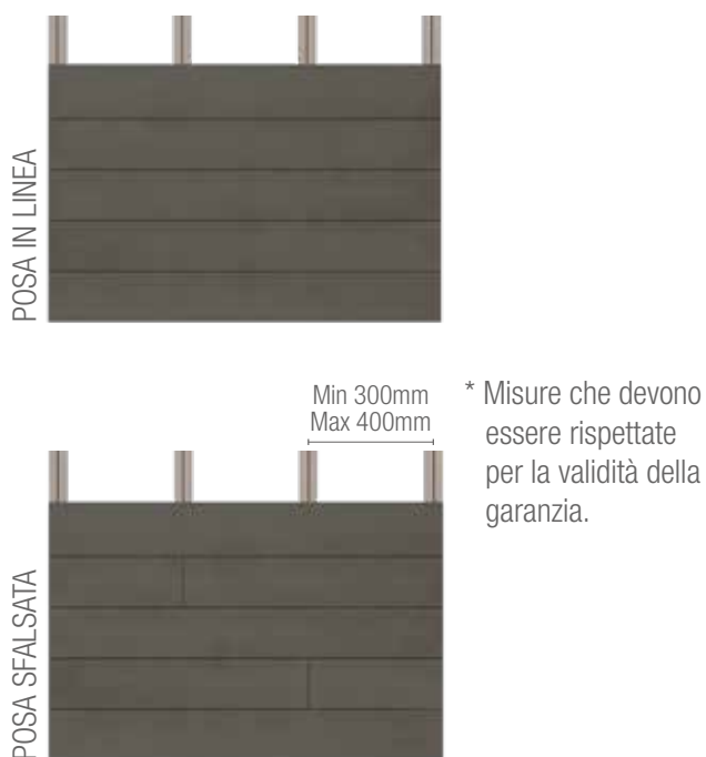
3.3 Posa orizzontale
